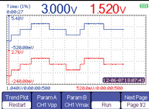
Экран регистратора (TREND PLOT в режиме Осциллограф)
