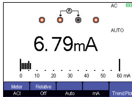
Экран регистратора (TREND PLOT в режиме Мультиметр)
